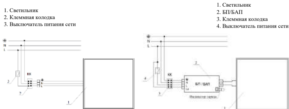
Рис. №3 Схема подключения светильника.
