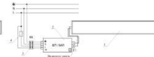
Рис. №3 Схема подключения светильника.
