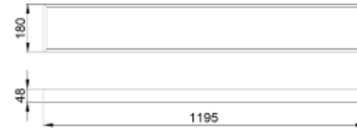
Рис.№1 Размеры светильника
