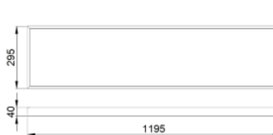
Рис.№1 Размеры светильника
