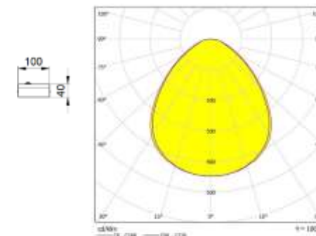
Рис.№2 Кривая силы света
