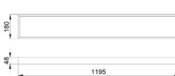
Рис.№1 Размеры светильника
