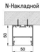
Длина светильника мм 475-2000
