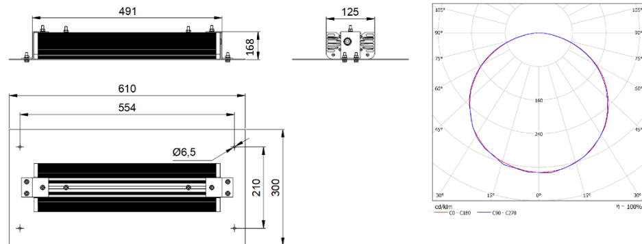
Рис.№1 Размеры светильника
