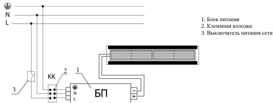
Рис. №3 Схема подключения светильника с драйвером к сети питания напряжения.
