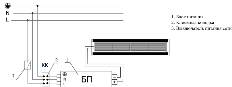
Рис. №3 Схема подключения светильника с драйвером к сети питания напряжения.
