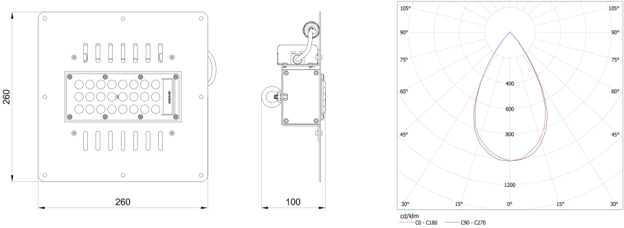
Рис.№1 Размеры светильника
