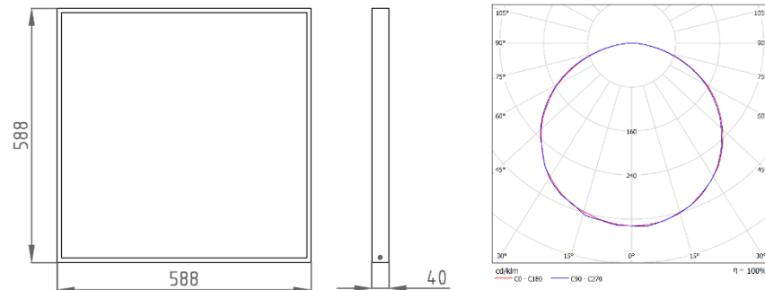
Рис.1 Размеры светильника
