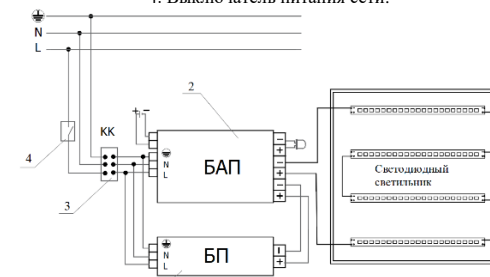
Рис. №4 Схема подключения светильника с БАП к сети питания напряжения.
