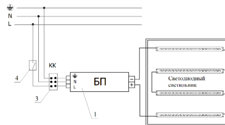
Рис. №3 Схема подключения светильника с драйвером к сети питания напряжения.
